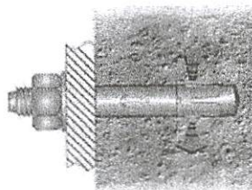
Sistema de Aperto de Chumbadores/Parafusos dentro do Concreto
